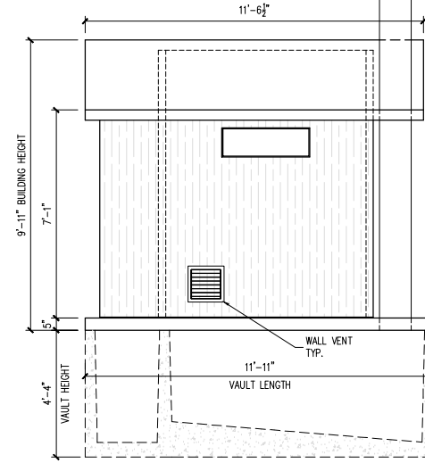
RIGHT ELEVATION
